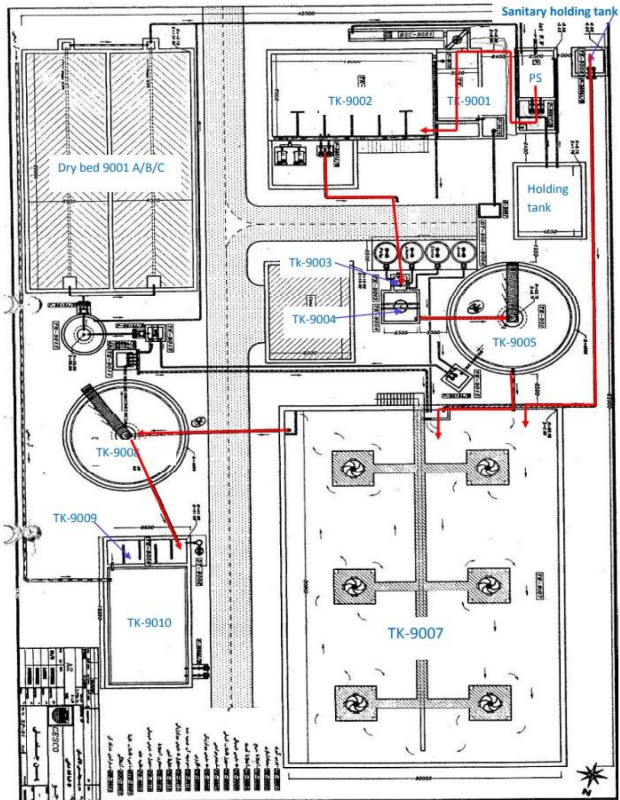
شکل شماره ۲- شماتیک واحد تصفیه خانه
