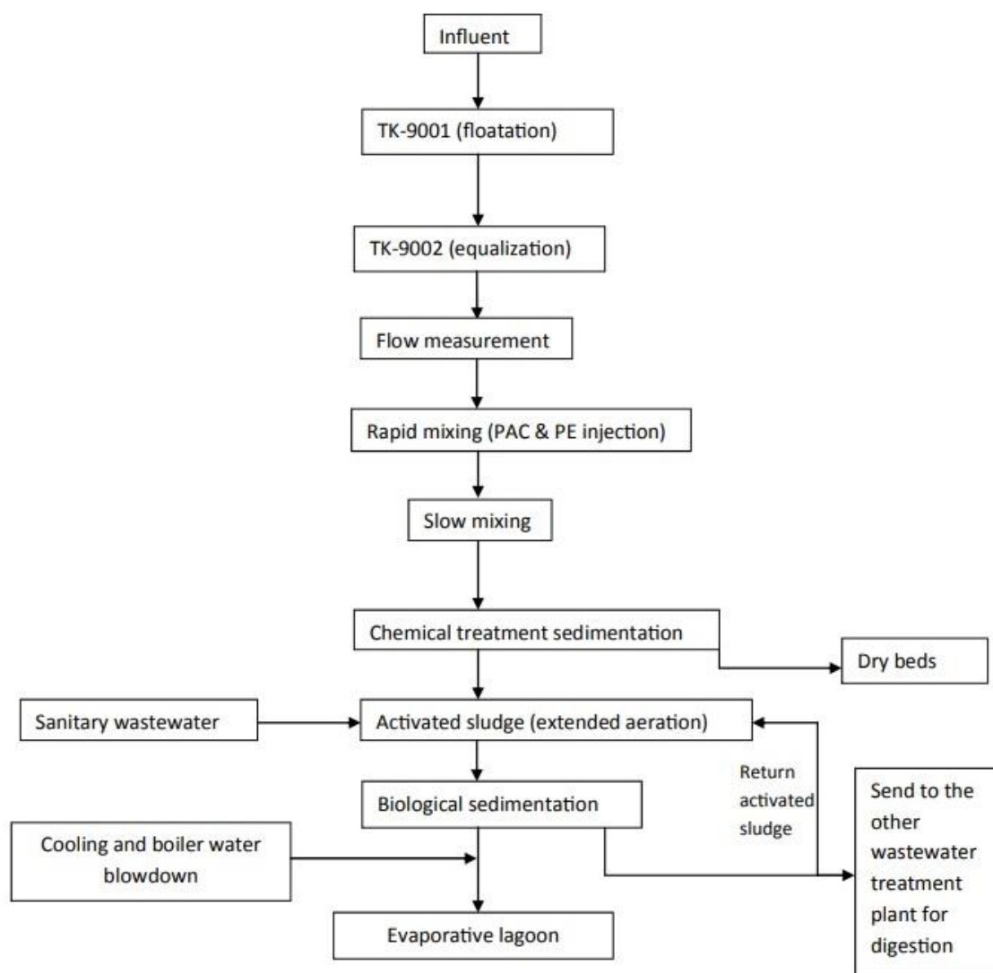
شکل شماره ۱- نمودار فرآیند واحد تصفیه خانه
